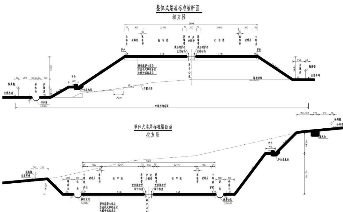
图 2.2 路基标准横断面图
