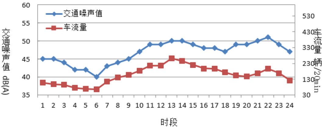
图 7.5 K373+010（路右）交通噪声 24 小时连续监测交通噪声监测值与车流量关系图
