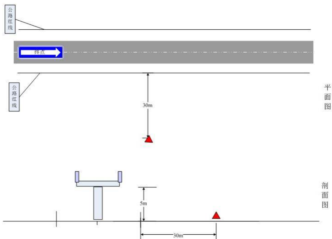
图 7.2 K373+010 (路右) 交通噪声 24 小时连续监测点位布设示意图
